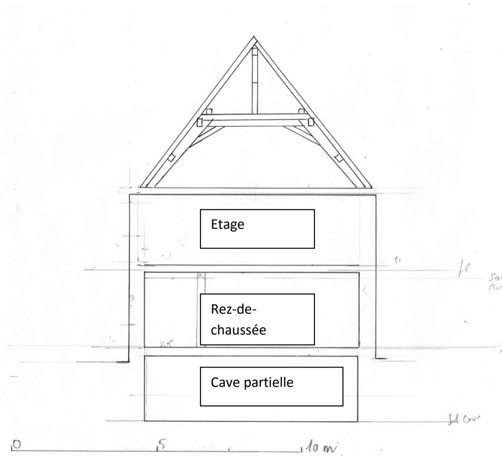
Figure 5. Coupe (provisoire) mettant en évidence le principe de charpente du toit
