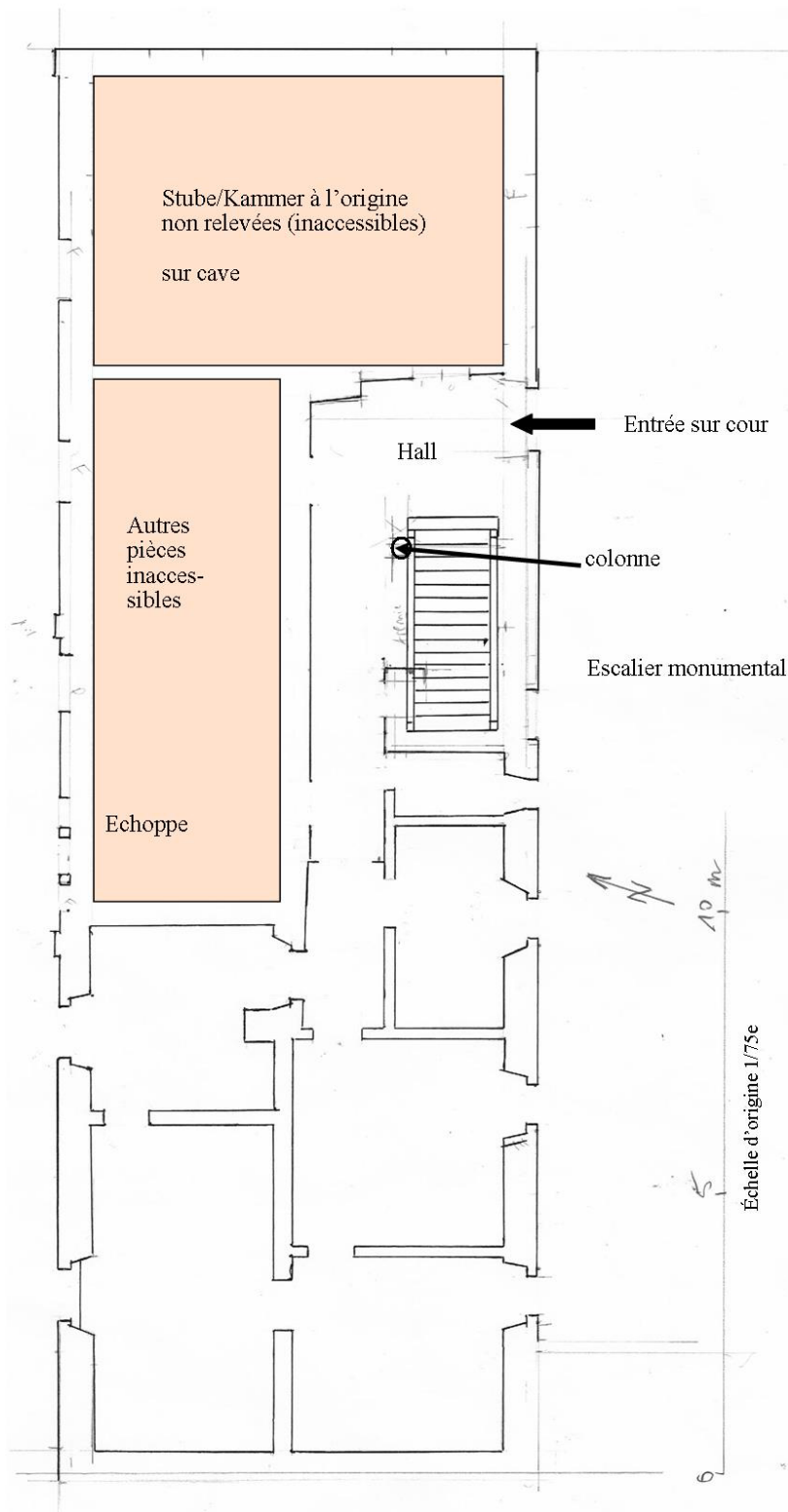
Figure 13. Plan sommaire du rez-de-chaussée (provisoire car l'accès à certaines pièces n'a pas été possible)
